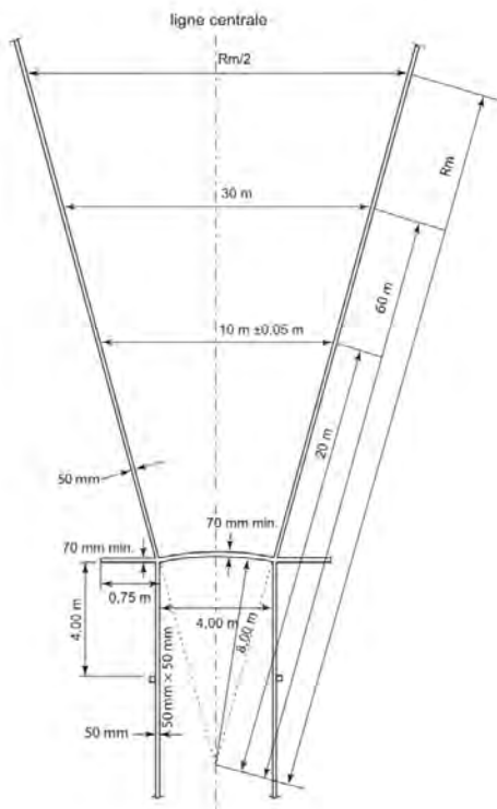
Schéma (e) RT32 (Règle 187) - Piste d'élán et secteur de chute pour le Lancer du javelot (pas à l'échelle)
