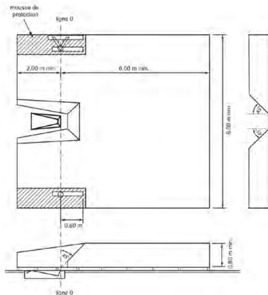
Schéma (c) RT28 (Règle 183) - Zone de réception du Saut à la perche (vue en plan et vue en coupe)
