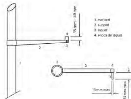
Schéma (b) RT28 (Règle 183) - Support de barre transversale (vue de la zone de réception et vue en plan)
